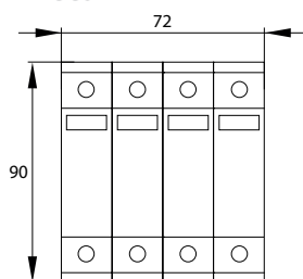
CCS02 - ogranicznik iskiernikowo warystorowy
