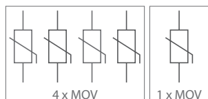
CCS01 - ogranicznik warystorowy
